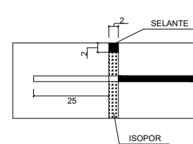
DETALHE DA JUNTA TRANSVERSAL DE EXPANSÃO
