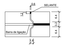
DETALHE DA JUNTA LONGITUDINAL
