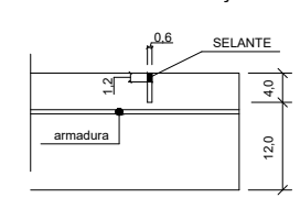
DETALHE DA JUNTA TRANSVERSAL DE RETRAÇÃO
